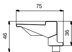
18a. Support du vitrage - FTP-V
