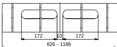
65b. Latte de l'entrée d'air - XHL - V2
