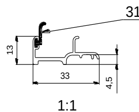
16a. Profilé d'aluminium FR041
