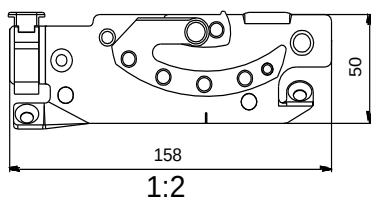
9. Ferrure - partie de l'ouvrant
