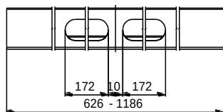
65a. Latte de l'entrée d'air - XHL - V1
