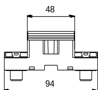
18a. Support du vitrage - FTP-V
