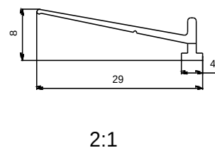
33. Joint supérieur BC230F
